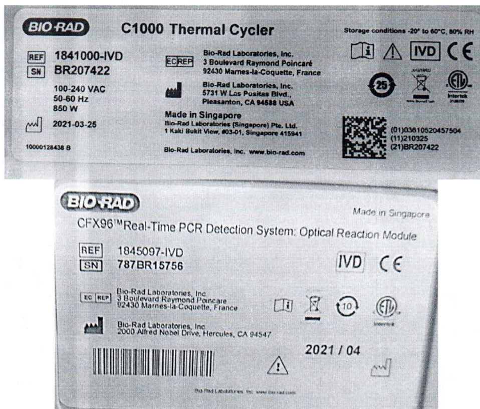
Рисунок 1.2 – Фотография маркировки термоциклера для амплификации нуклеиновых кислот модель C1000 Thermal Cycler № BR207422 с модулем оптическим реакционным CFX96™ № 787BR15756
