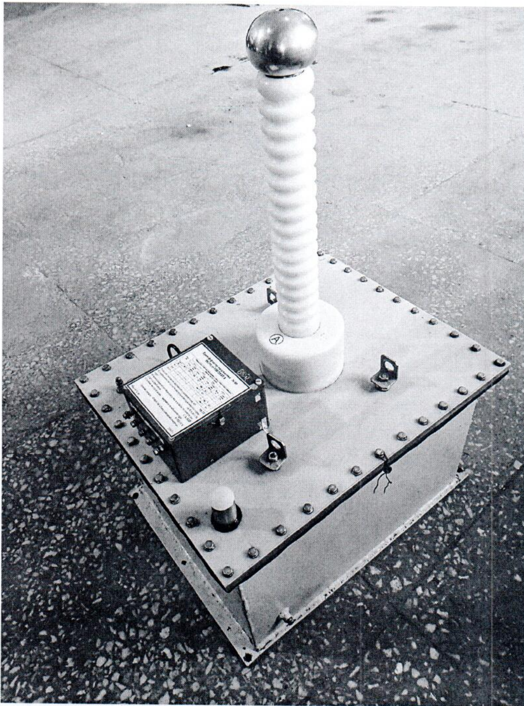
Рисунок 1.1 – Фотография общего вида трансформатора напряжения НОМ(э)-110/35/27,5 № 05
