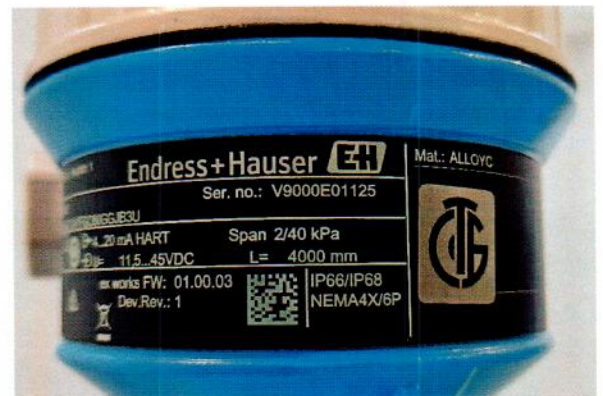
Рисунок 1.3 – Фотографии маркировки преобразователя
