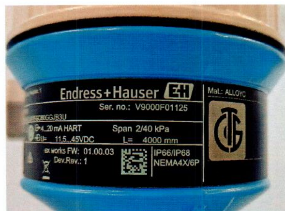
Рисунок 1.3 – Фотографии маркировки преобразователя
