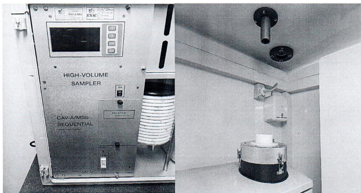
Рисунок 1.1 – Фотографии общего вида высокочастотного пробоотборника твердых частиц CAV-A/MSb № В-144/0160
