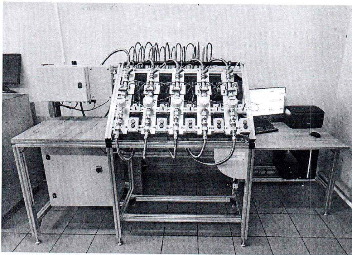
Рисунок 1.1 – Фотография общего вида установки для поверки счетчиков газа ПОТОК УПСГ-12 № 012
