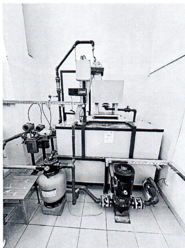
Рисунок 1.1 – Фотографии общего вида установки проливной расходомерной «Поток 5.025» № 011
