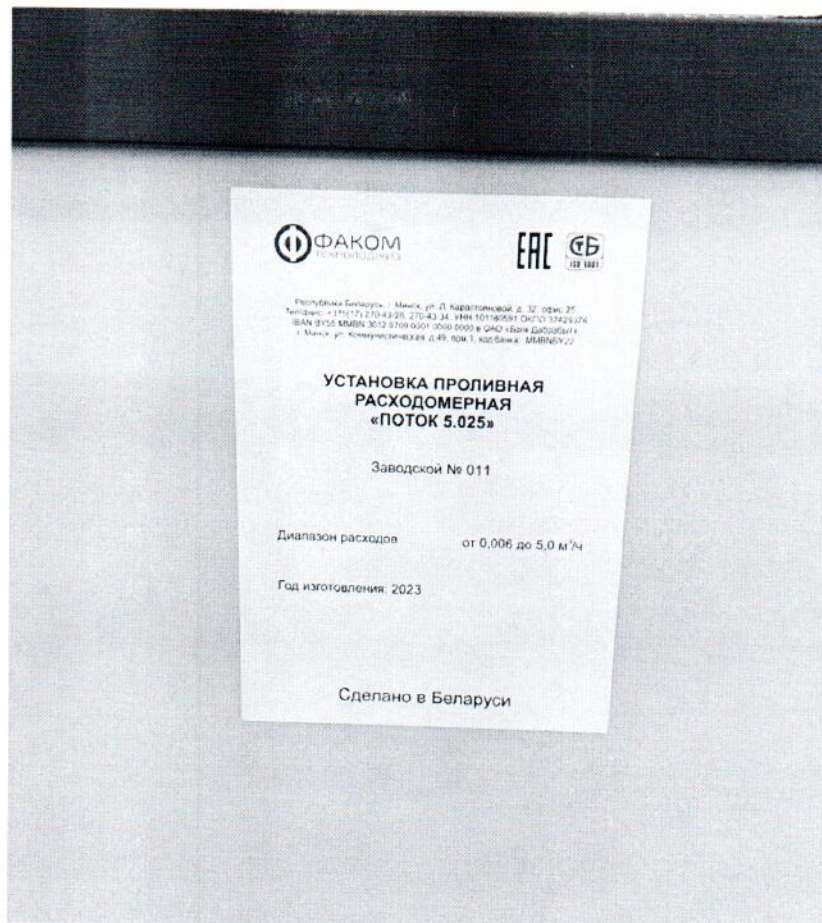
Рисунок 1.2 – Фотография маркировки установки проливной расходомерной «Поток 5.025» № 011
