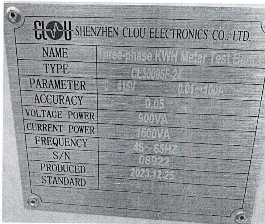
Рисунок 1.2 – Фотография маркировки установки для поверки счётчиков электрической энергии CL30005F-24, зав.№ 08922. (изображение носит иллюстративный характер)
