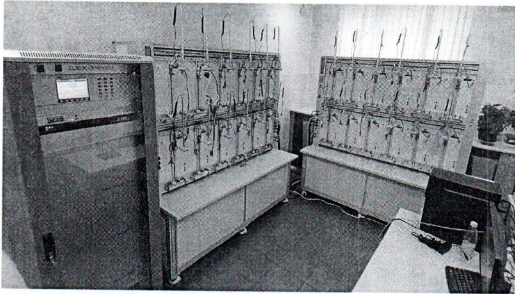
Рисунок 1.1 – Фотография общего вида установки для поверки счётчиков электрической энергии CL30005F-24, зав.№ 08922. (изображение носит иллюстративный характер)
