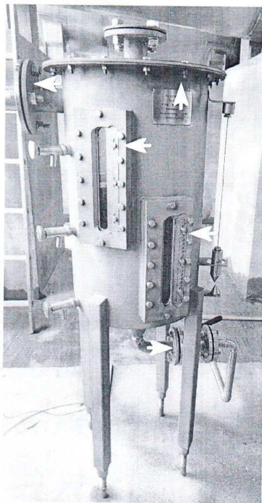
Рисунок 3.1 – Места пломбировки от несанкционированного доступа
