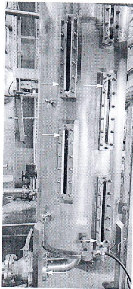
Рисунок 3.2 – Схема пломбировки шкальных пластин и фланца сливного патрубка от несанкционированного доступа
