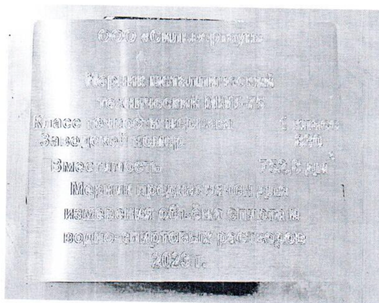
Рисунок 1.2 – Внешний вид маркировочной таблички мерника металличе- ского технического ММТ-75 № 830
