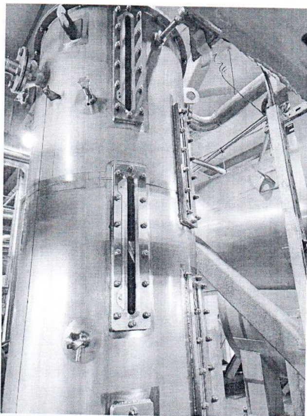
Рисунок 1.1 – Внешний вид мерника металлического технического ММТ-75 № 830
