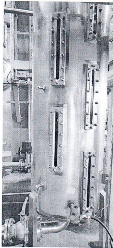
Рисунок 1.1 – Внешний вид мерника металлического технического ММТ-75 № 832
