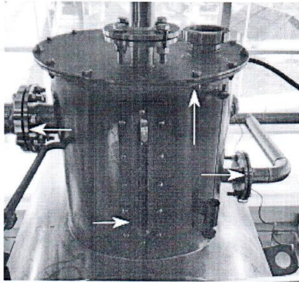
Рисунок 3.1 – Схема пломбировки крышки-фланца, фланцев наливной и переливной труб и шкальной пластины от несанкционированного доступа
