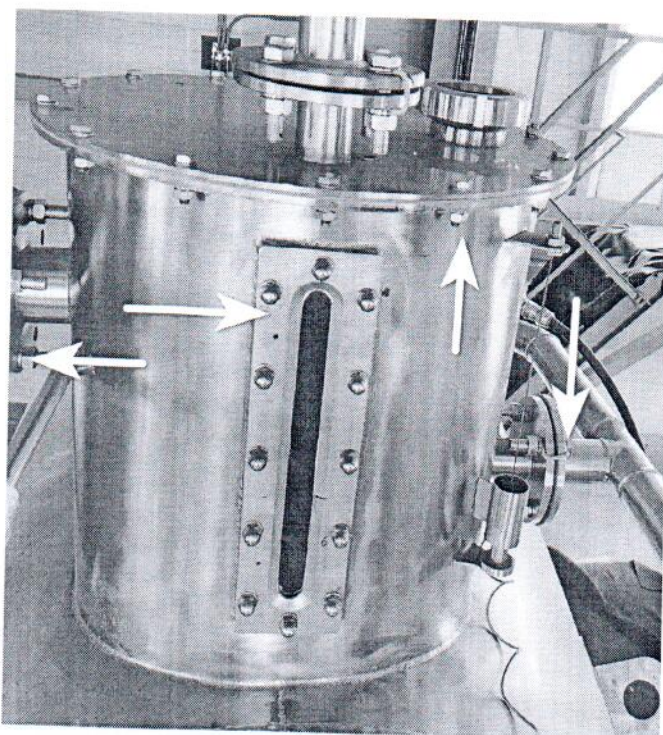
Рисунок 3.1 – Схема пломбировки крыши-фланца, фланцев наливной и переливной труб и шкальной пластины от несанкционированного доступа
