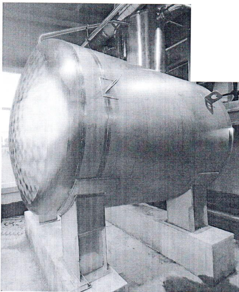
Рисунок 1.1 – Внешний вид мерника металлического технического ММТ-1000 № 838
