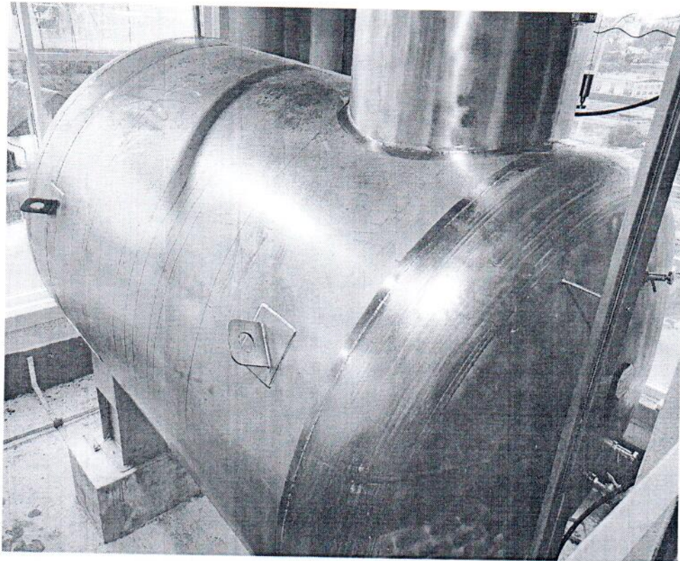
Рисунок 1.1 – Внешний вид мерника металлического технического ММТ-1000 № 840
