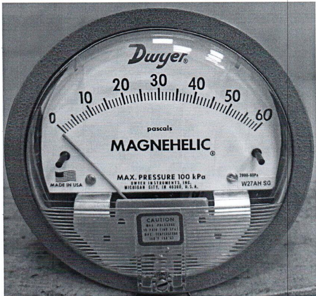
Рисунок 1.1 – Фотография общего вида манометра дифференциального показывающего Magnehelic 2000-60PA № 161222СК-37
