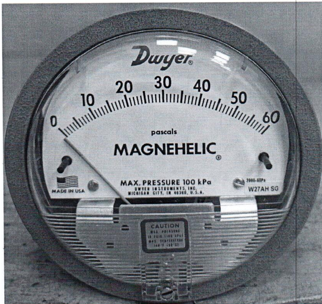
Рисунок 1.1 – Фотография общего вида манометра дифференциального показывающего Magnehelic 2000-60РА № 161222СК-36
