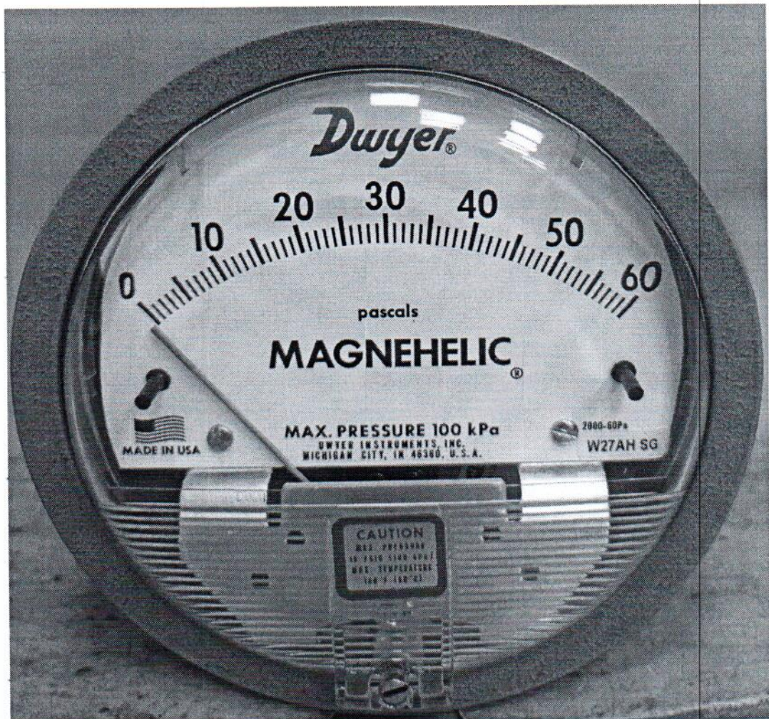
Рисунок 1.1 – Фотография общего вида манометра дифференциального показывающего Magnehelic 2000-60РА № 161222СК-35
