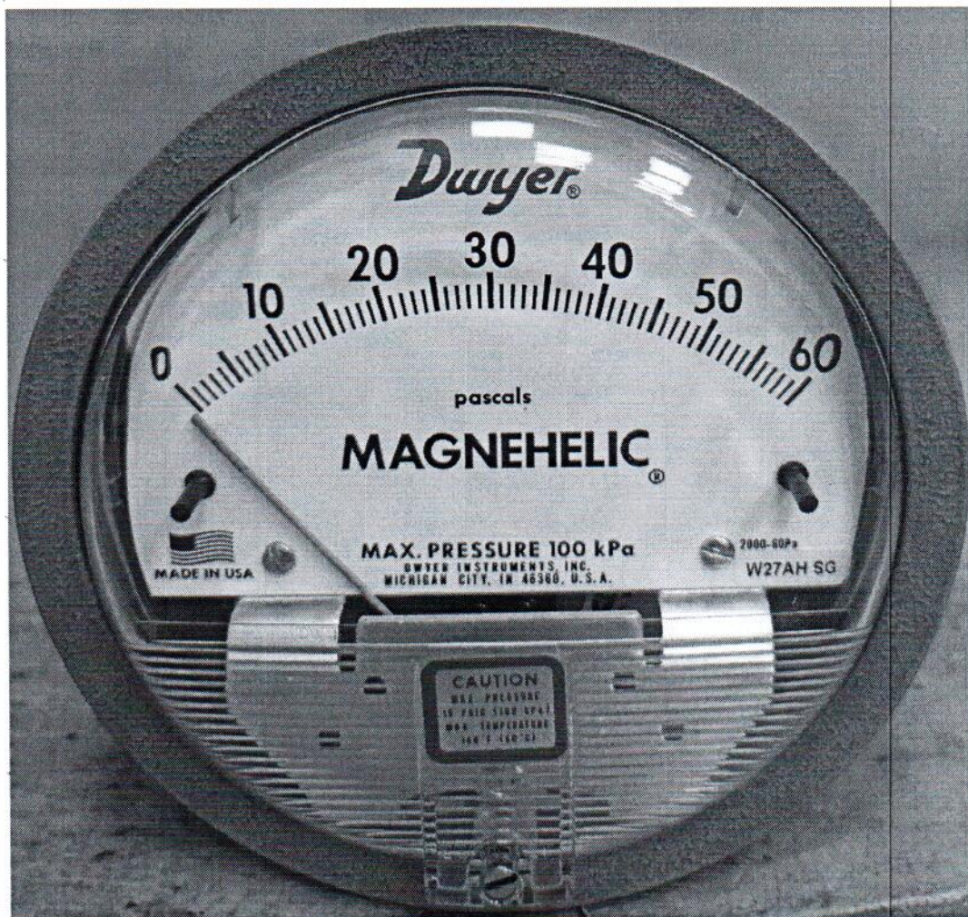
Рисунок 1.1 – Фотография общего вида манометра дифференциального показывающего Magnehelic 2000-60PA № 161222СК-34
