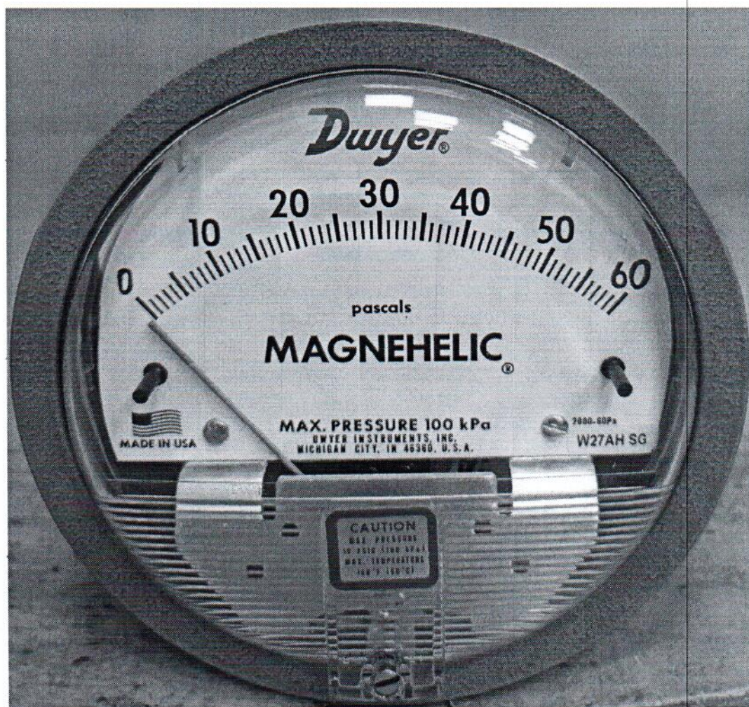
Рисунок 1.1 – Фотография общего вида манометра дифференциального показывающего Magnehelic 2000-60PA № 161222СК-33
