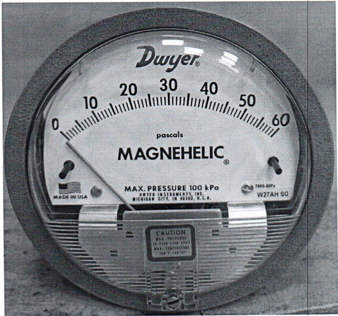
Рисунок 1.1 – Фотография общего вида манометра дифференциального показывающего Magnehelic 2000-60РА № 161222СК-32
