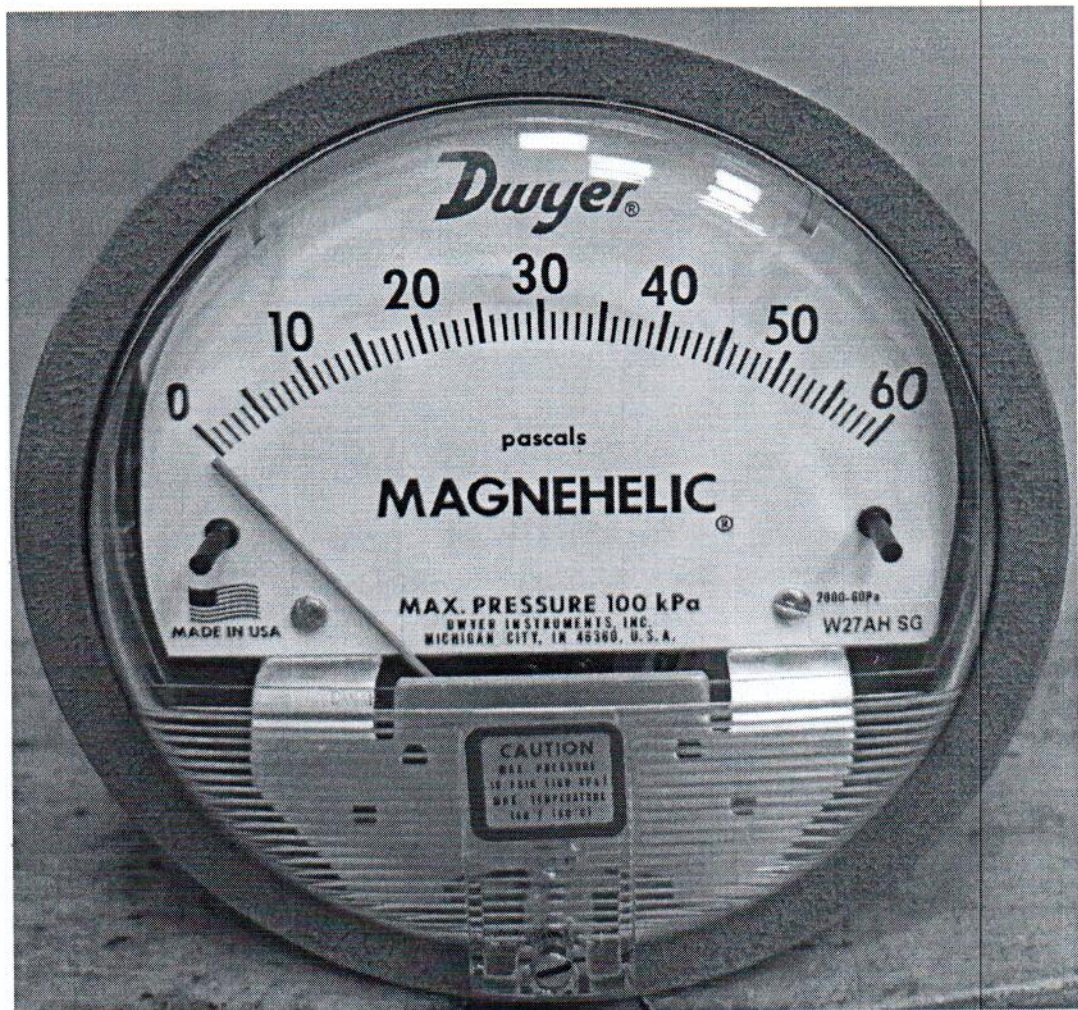
Рисунок 1.1 – Фотография общего вида манометра дифференциального показывающего Magnehelic 2000-60РА № 161222СК-31
