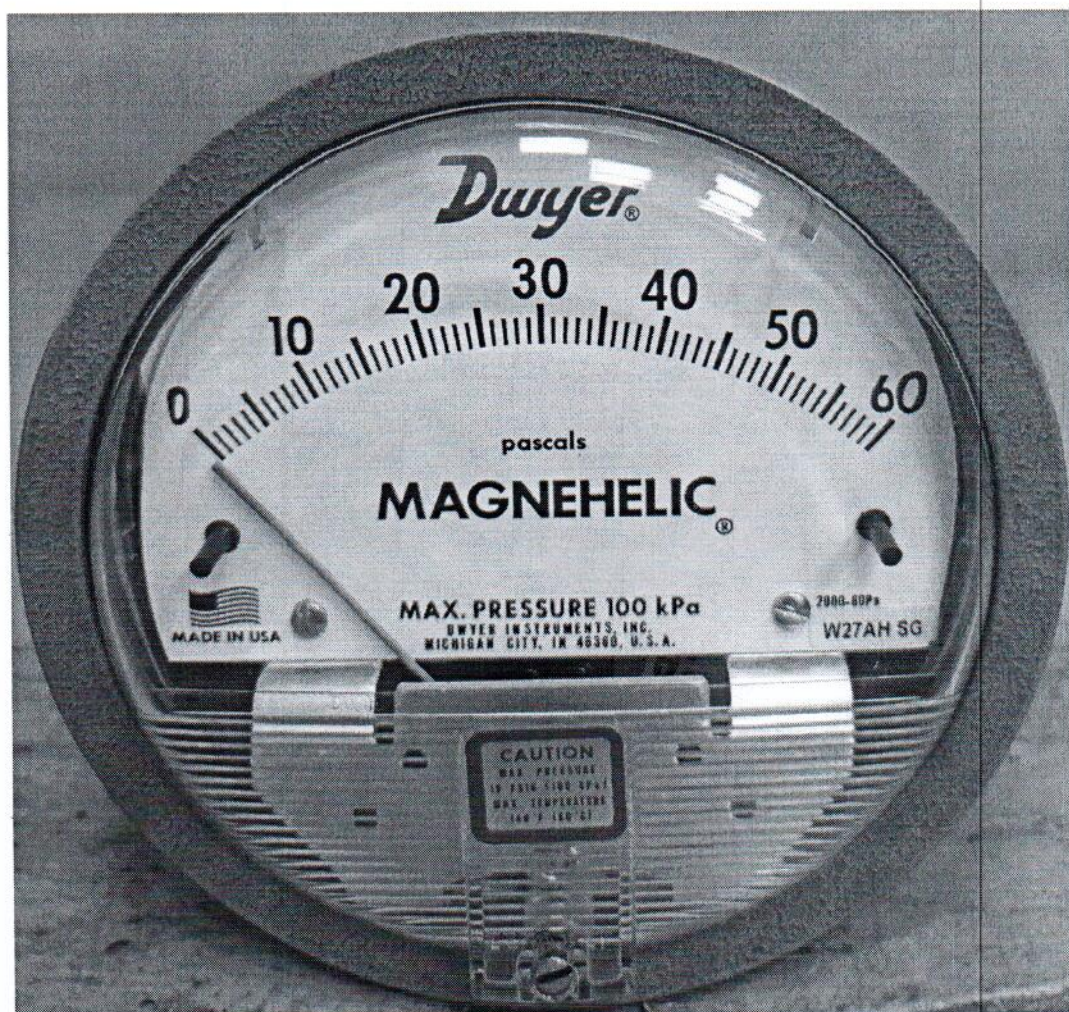
Рисунок 1.1 – Фотография общего вида манометра дифференциального показывающего Magnehelic 2000-60РА № 161222СК-30
