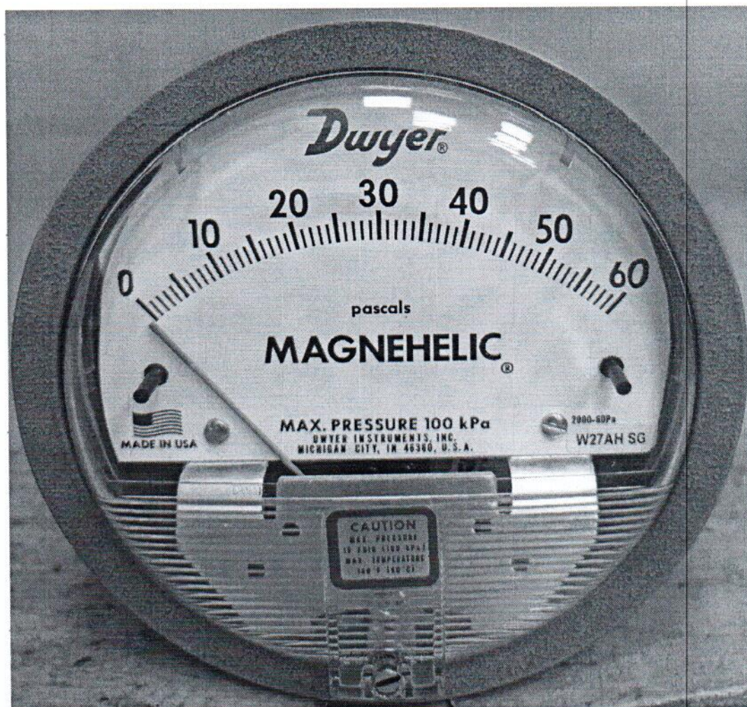
Рисунок 1.1 – Фотография общего вида манометра дифференциального показывающего Magnehelic 2000-60РА № 161222СК-26
