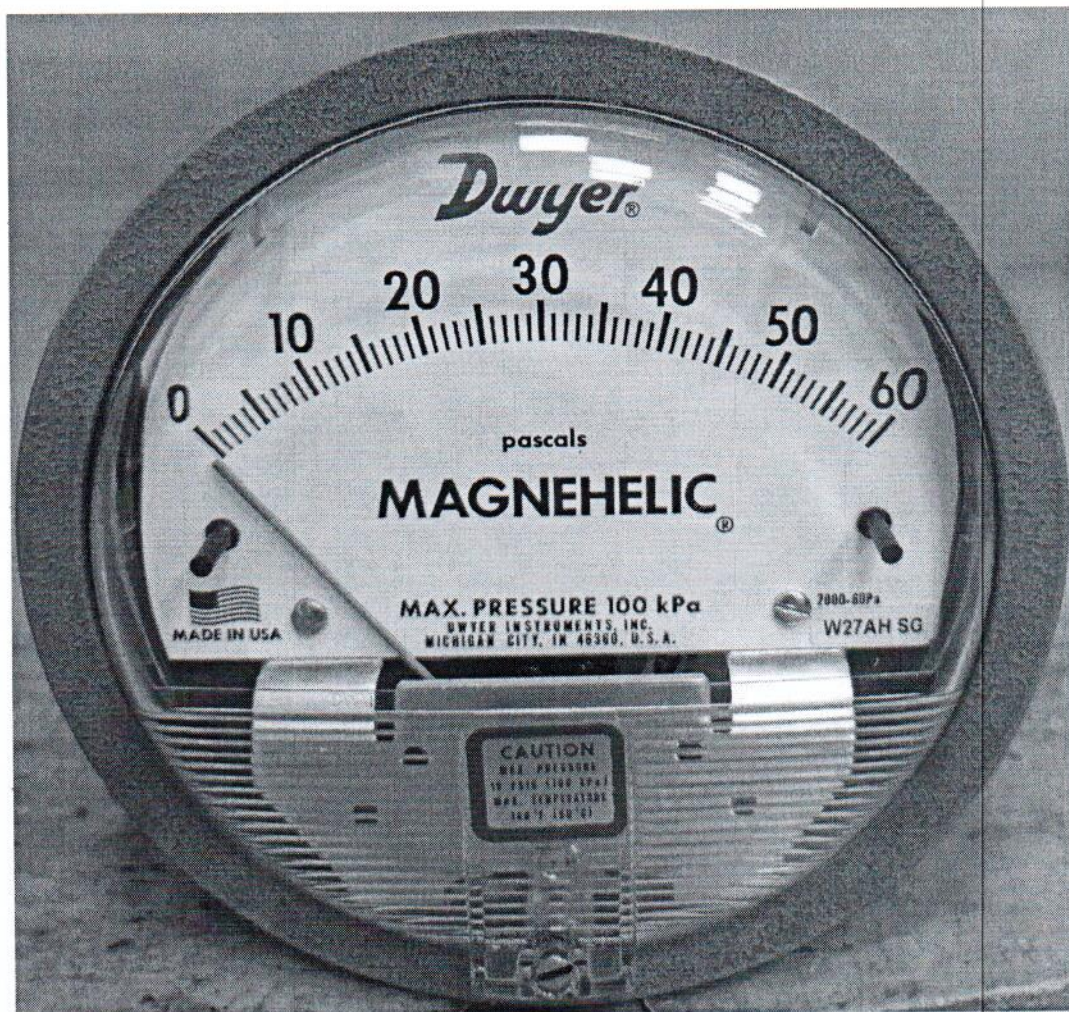
Рисунок 1.1 – Фотография общего вида манометра дифференциального показывающего Magnehelic 2000-60РА № 161222СК-25
