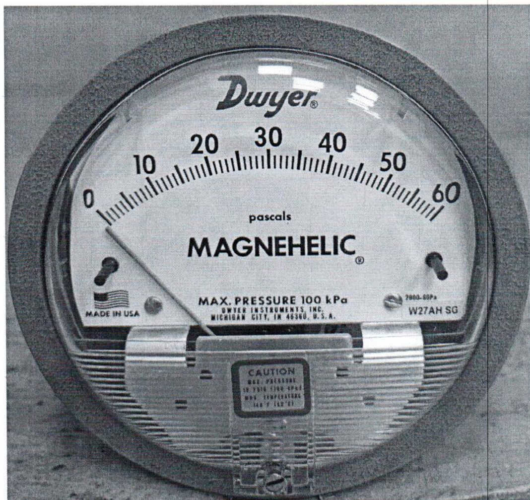
Рисунок 1.1 – Фотография общего вида манометра дифференциального показывающего Magnehelic 2000-60PA № 161222СК-24
