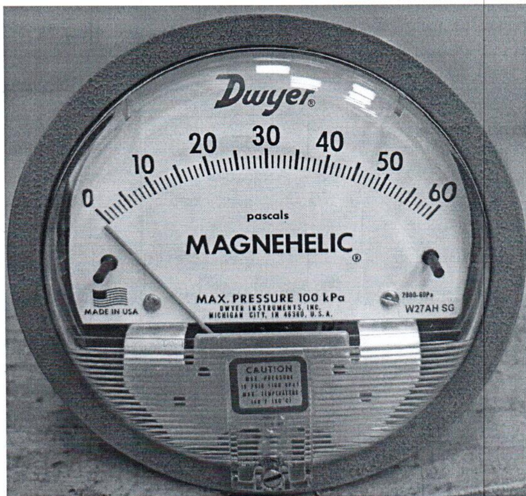
Рисунок 1.1 – Фотография общего вида манометра дифференциального показывающего Magnehelic 2000-60PA № 161222СК-22
