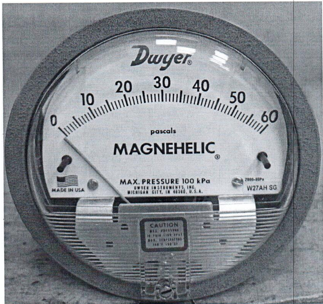
Рисунок 1.1 – Фотография общего вида манометра дифференциального показывающего Magnehelic 2000-60РА № 161222СК-19
