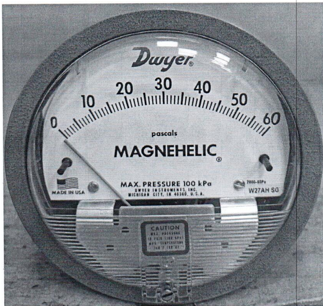
Рисунок 1.1 – Фотография общего вида манометра дифференциального показывающего Magnehelic 2000-60PA № 161222СК-17
