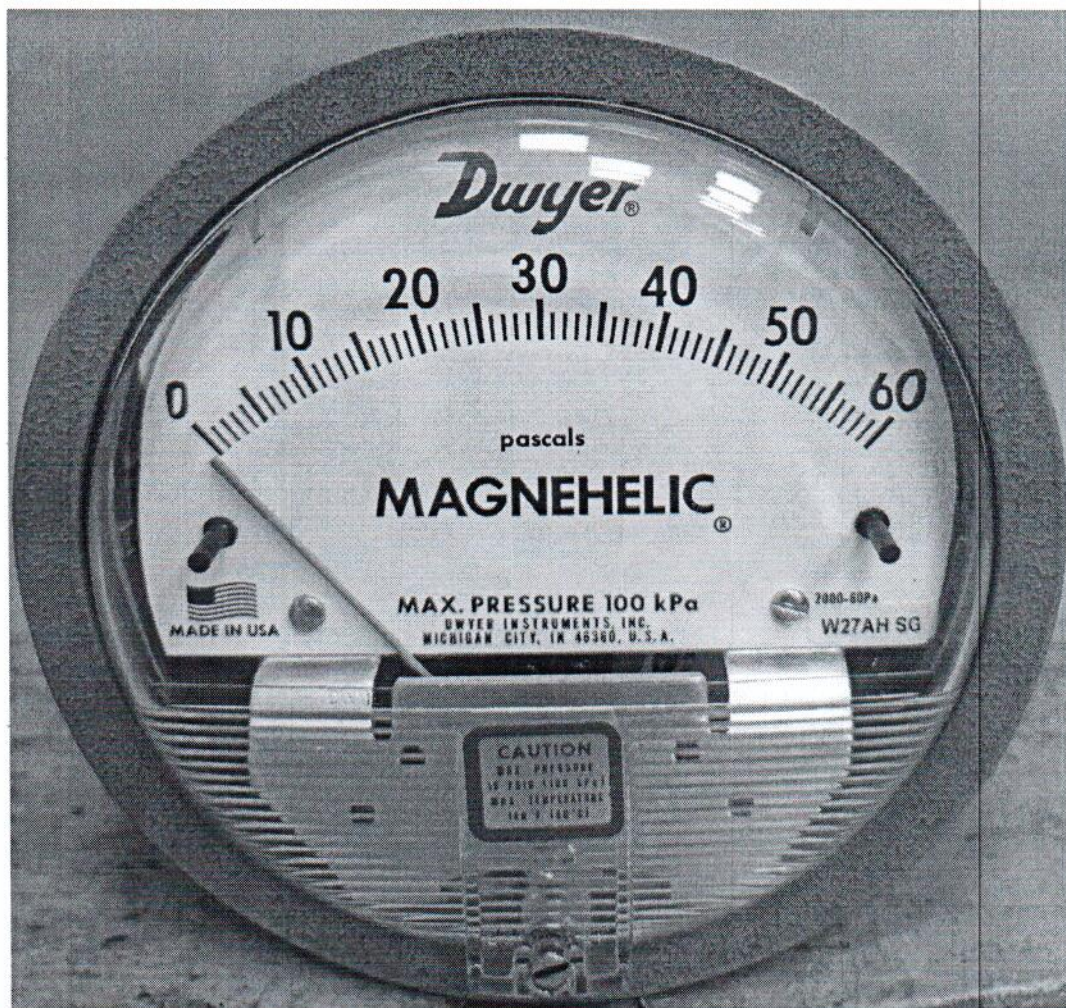
Рисунок 1.1 – Фотография общего вида манометра дифференциального показывающего Magnehelic 2000-60PA № 161222СК-16
