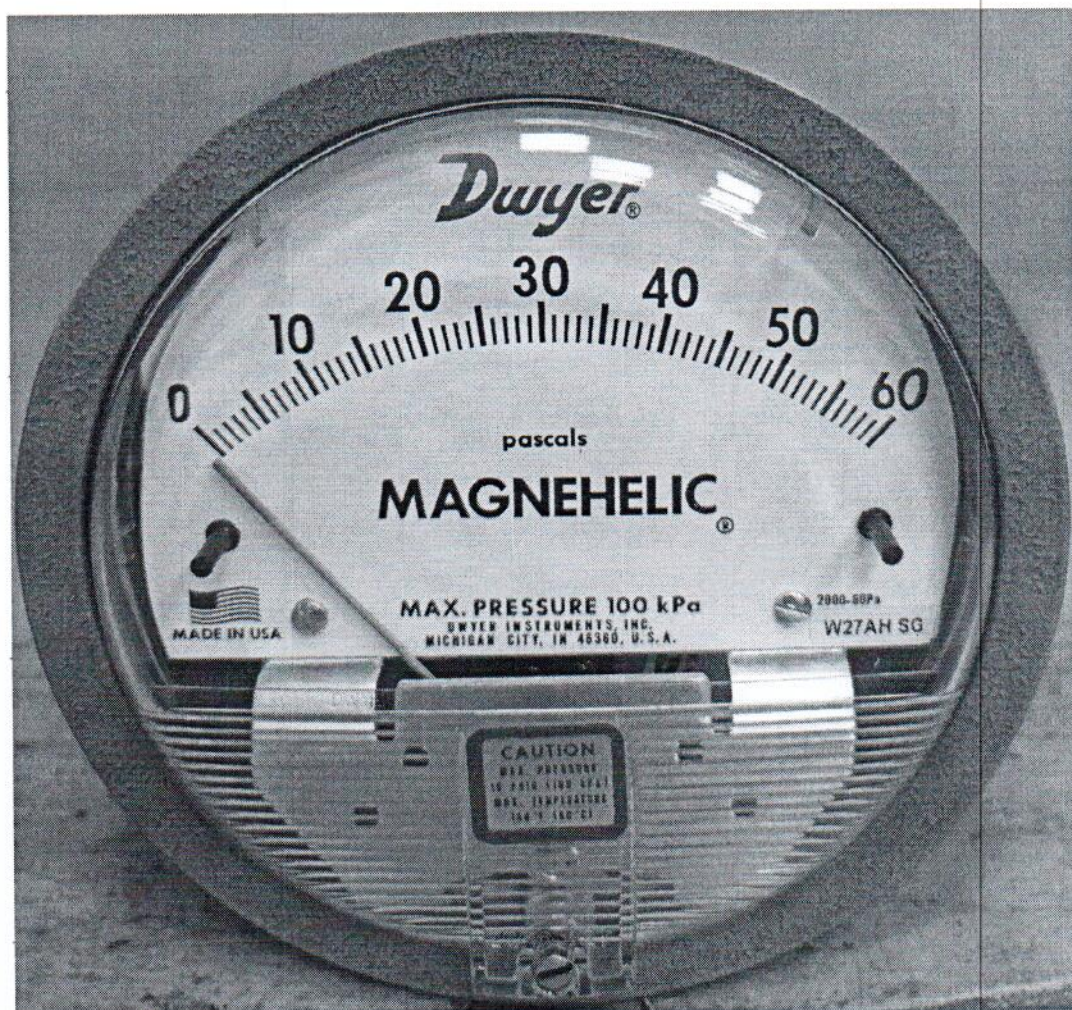
Рисунок 1.1 – Фотография общего вида манометра дифференциального показывающего Magnehelic 2000-60PA № 161222СК-15
