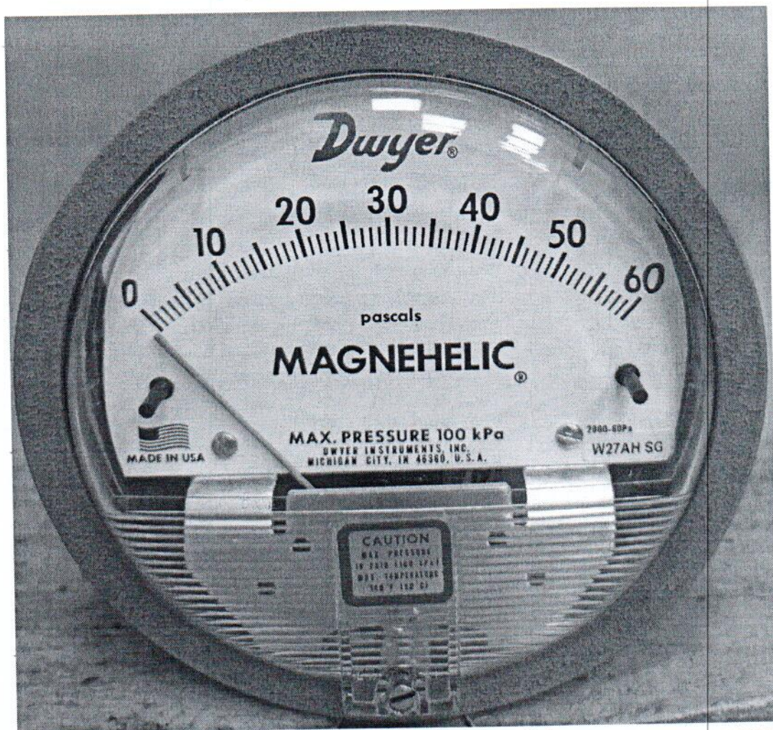
Рисунок 1.1 – Фотография общего вида манометра дифференциального показывающего Magnehelic 2000-60PA № 161222СК-13
