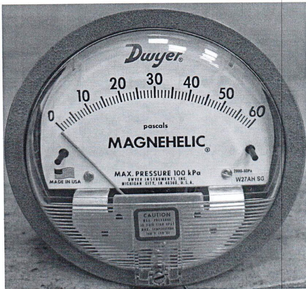
Рисунок 1.1 – Фотография общего вида манометра дифференциального показывающего Magnehelic 2000-60PA № 161222СК-12
