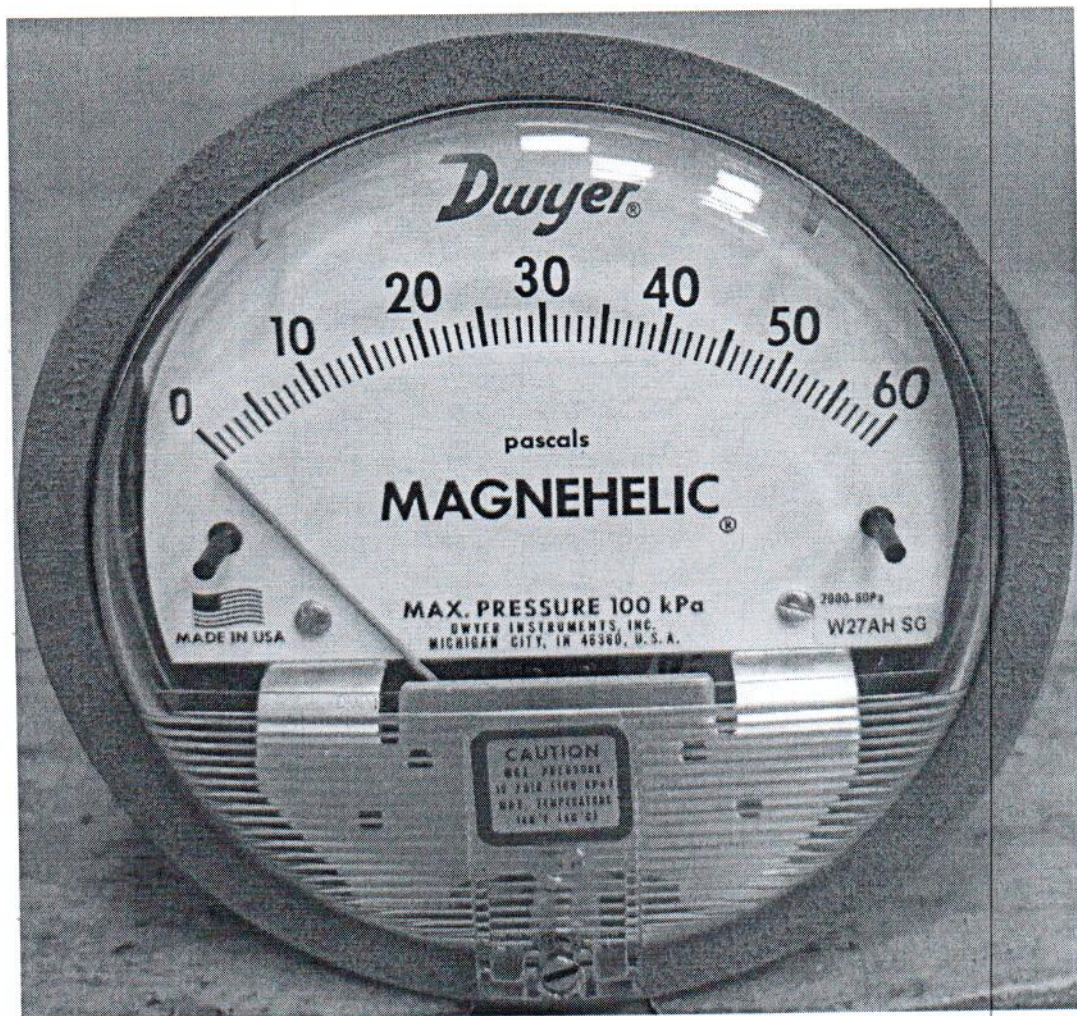
Рисунок 1.1 – Фотография общего вида манометра дифференциального показывающего Magnehelic 2000-60РА № 161222СК-11
