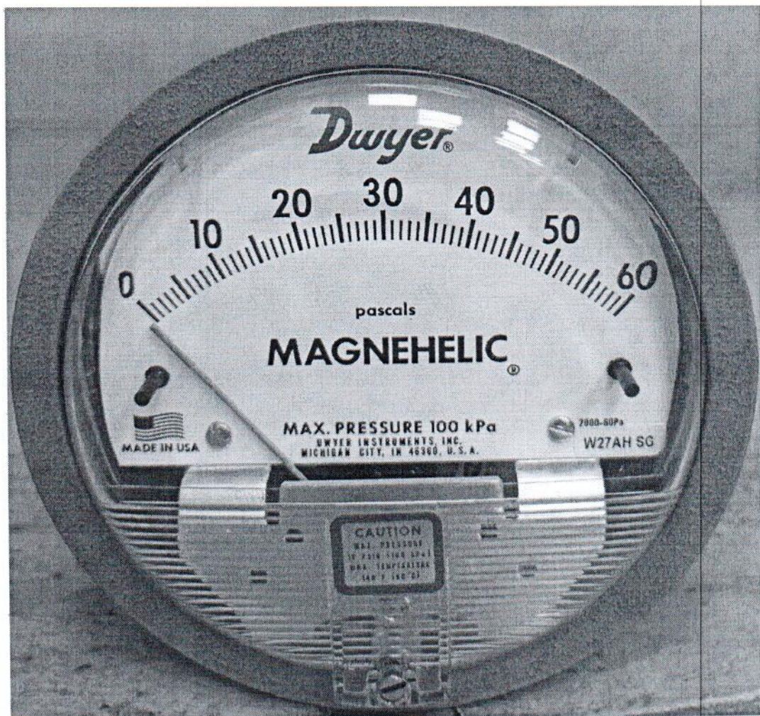
Рисунок 1.1 – Фотография общего вида манометра дифференциального показывающего Magnehelic 2000-60PA № 161222СК-10
