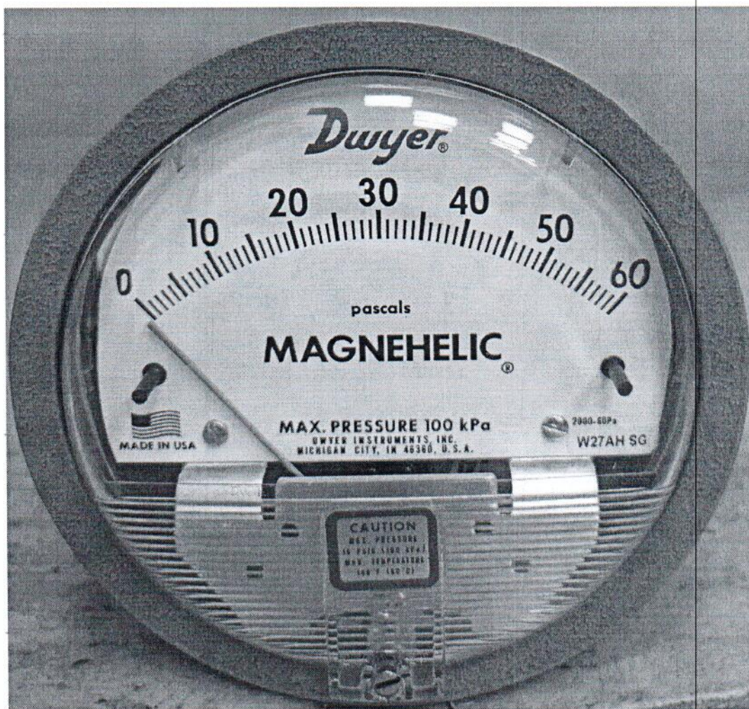
Рисунок 1.1 – Фотография общего вида манометра дифференциального показывающего Magnehelic 2000-60РА № 161222СК-06
