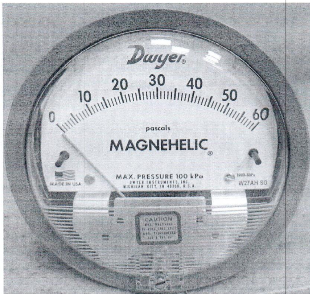
Рисунок 1.1 – Фотография общего вида манометра дифференциального показывающего Magnehelic 2000-60РА № 161222СК-04
