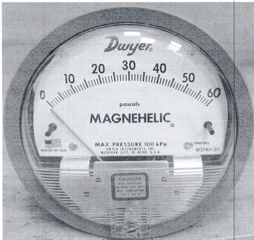
Рисунок 1.1 – Фотография общего вида манометра дифференциального показывающего Magnehelic 2000-60PA № 161222СК-03
