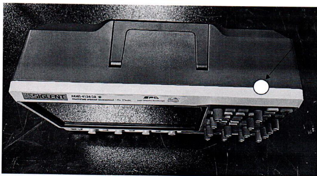
Рисунок 2.1 – Место нанесения знака поверки осциллографа цифрового запоминающего АКМП-4134/3А № SDS5XB0Q7R0707
