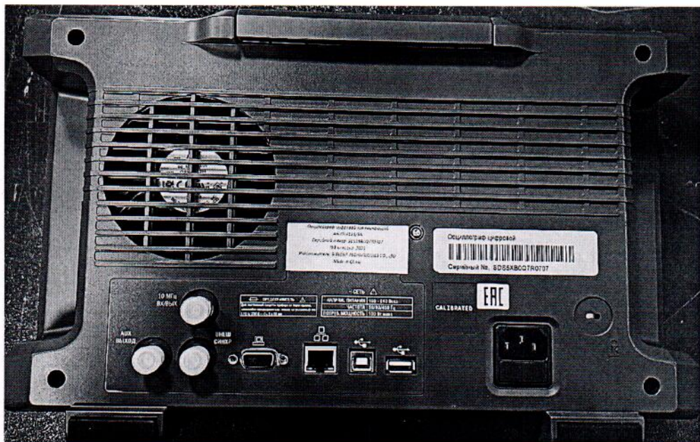
Рисунок 1.2 – Фотография задней панели осциллографа цифрового запоминающего АКИП-4134/3А № SDS5XB0Q7R0707
