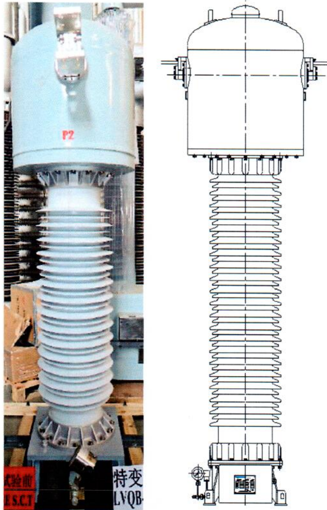
Рисунок 1.1 – Внешний вид трансформаторов тока измерительных элегазовых LWQB (изображение носит иллюстративный характер)
