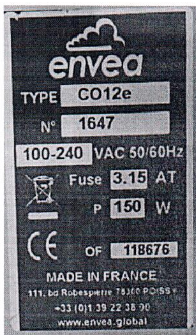
Рисунок 1.2 – Фотография маркировки газоанализатора CO12e № 1647
