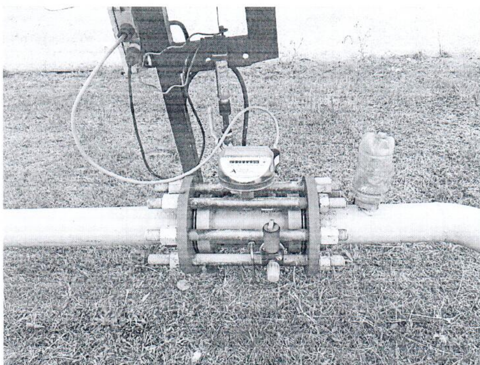
Рисунок 1.1 – Фотографии общего вида ИС УИГ
