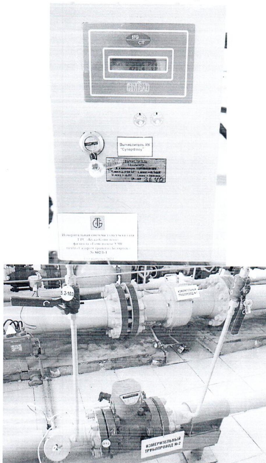
Рисунок 1.1 – Фотографии общего вида ИС УУГ
