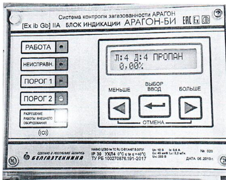
Рисунок 1.3 – Фотография маркировки блока индикации АРАГОН-БИ (изображение носит иллюстративный характер)
