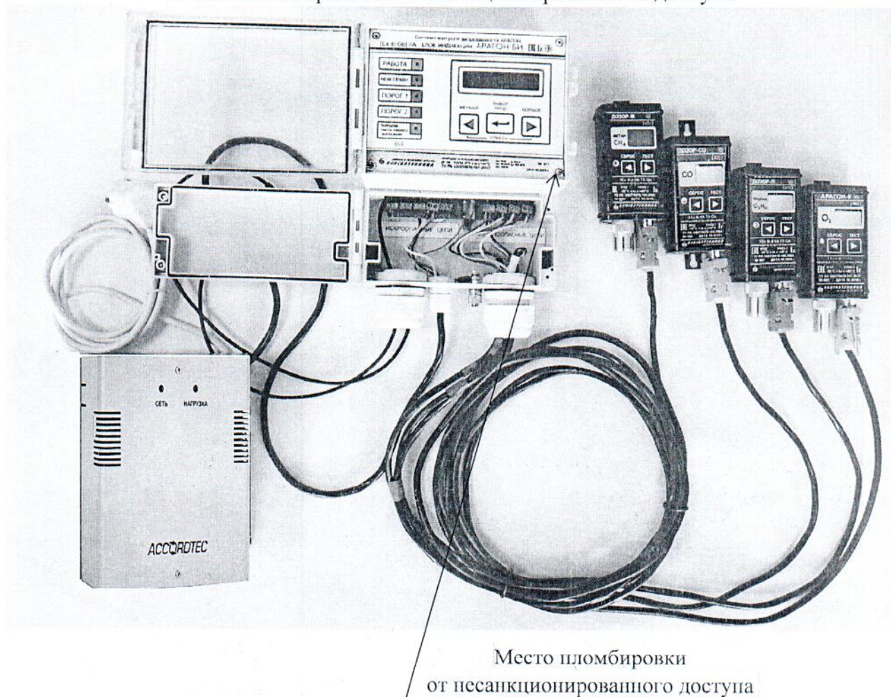
Рисунок 3.1 – Схема пломбировки от несанкционированного доступа
