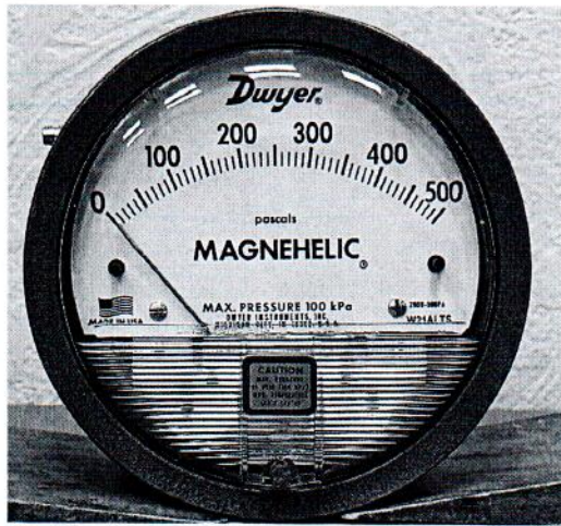
Рисунок 1.1 – Фотография общего вида манометра дифференциального показывающего Magnehelic 2000-500PA № 1302723СК-39
