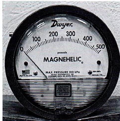
Рисунок 1.1 – Фотография общего вида манометра дифференциального показывающего Magnehelic 2000-500РА № 1302723СК-37
