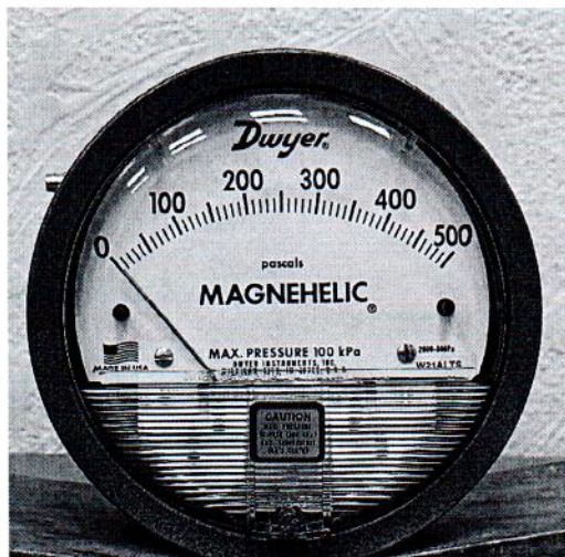
Рисунок 1.1 – Фотография общего вида манометра дифференциального показывающего Magnehelic 2000-500PA № 1302723СК-31
