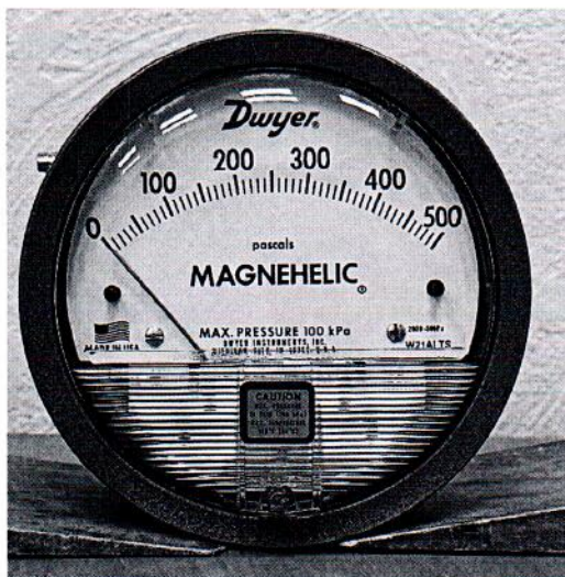
Рисунок 1.1 – Фотография общего вида манометра дифференциального показывающего Magnehelic 2000-500PA № 1302723СК-40
