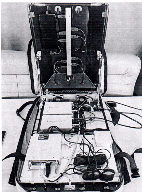
Рисунок 1.1 – Фотографии общего вида носимого измерительного комплекса для анализа параметров качества обслуживания сетей связи R&S Freerider 4 № 103411
