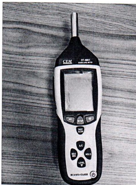
Рисунок 1.1 – Фотография общего вида измерителя уровня звука DT- 8852 № 150301778
