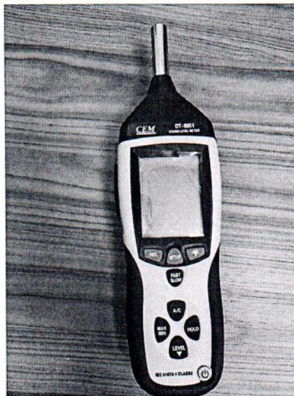
Рисунок 1.1 – Фотография общего вида измерителя уровня звука DT- 8851 № 12044637
